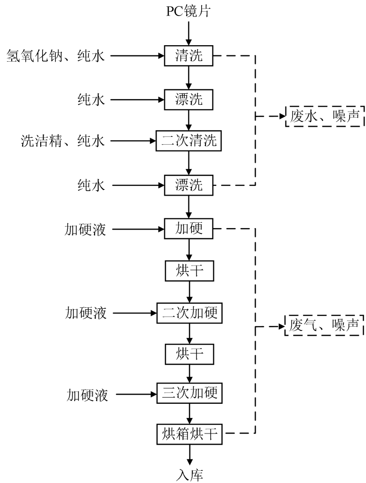
图 2-2 PC 镜片生产工艺流程及产污环节示意图
