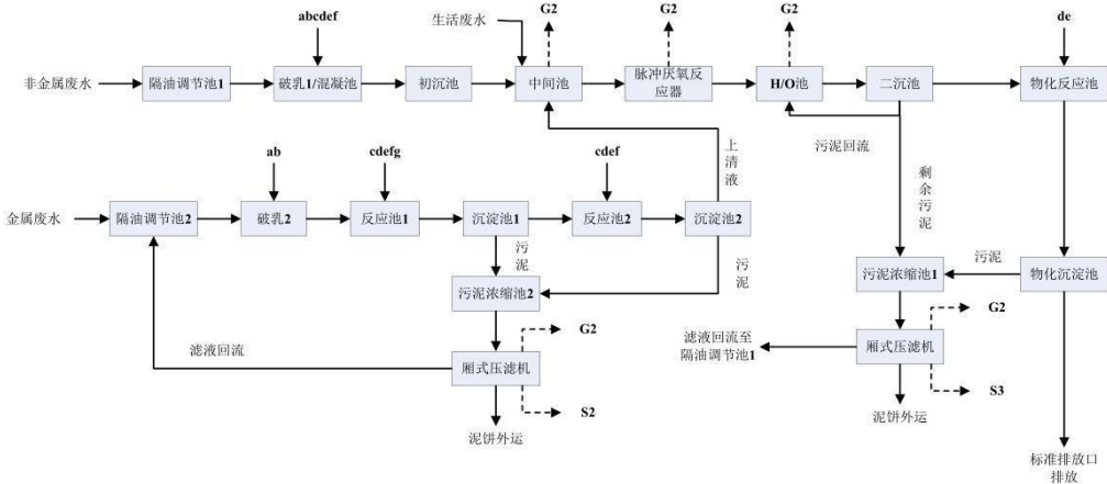
图 4-1 瑞安市马屿镇时代创业园污水处理站废水处理工艺流程图
