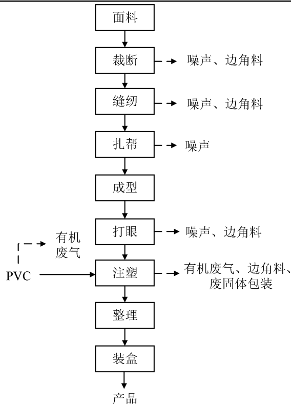
图 2-2 注塑鞋生产工艺
